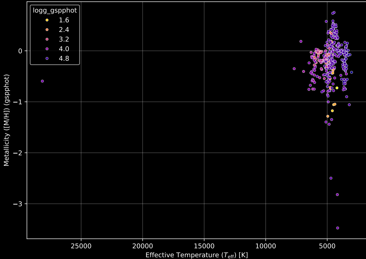
APOGEE DR17 Field: [270+75] Stellar Population Parameters (n= 381)
